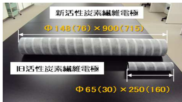
図5 新電極と旧電極
