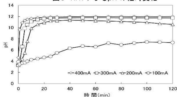
図4 電流によるpHの経時変化(既往研究)
