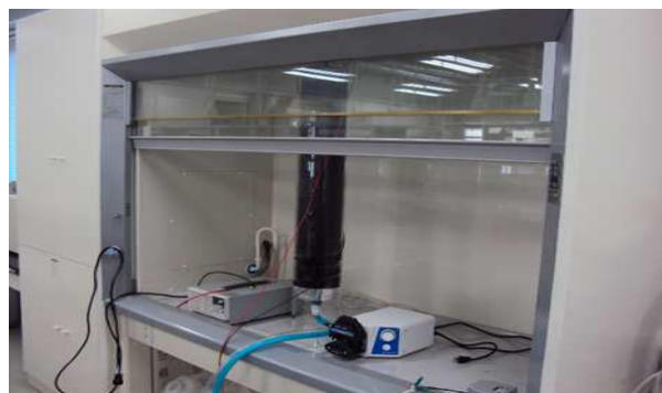
図6 ベンチスケールの通電システム
