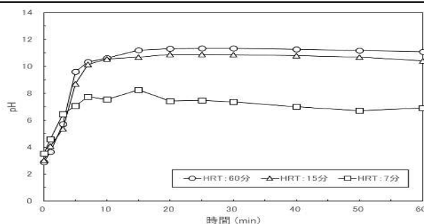
図3 HRTによるpHの経時変化
